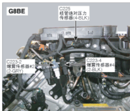
62. 发动机后部
