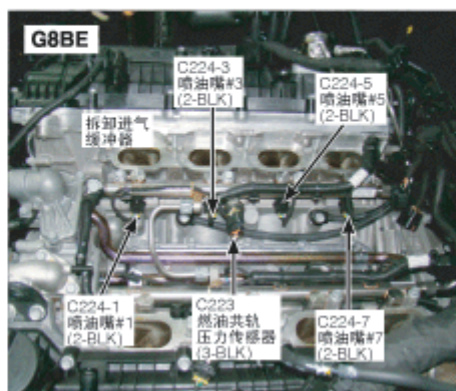
65. 发动机顶部
