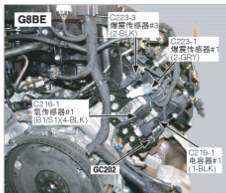
63. 发动机后右
