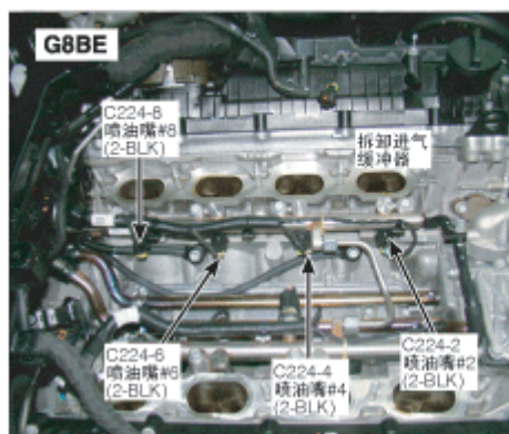
64. 发动机顶部
