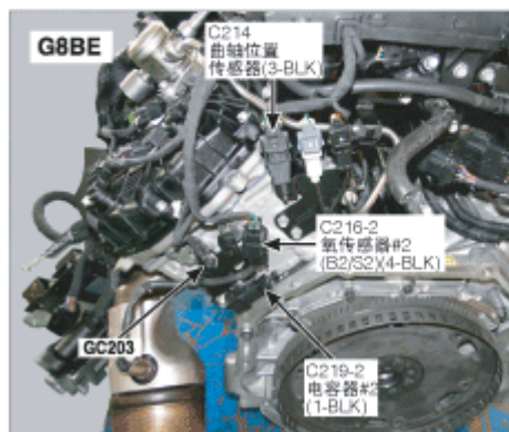
61. 发动机后左
