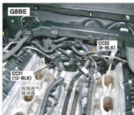
66. 发动机后部
